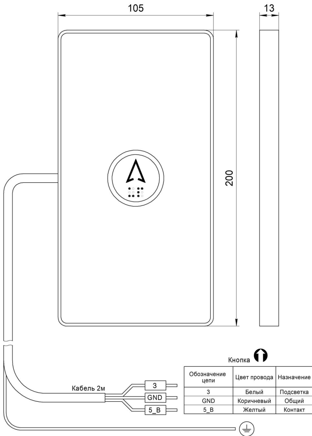
Рис.1 Внешний вид и габаритные размеры Вызывного поста МАЛАХИТ НШЕК.468381.061
